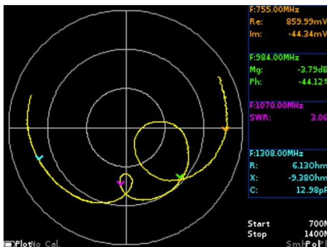
Рисунок 10.2 – Полярная диаграмма
